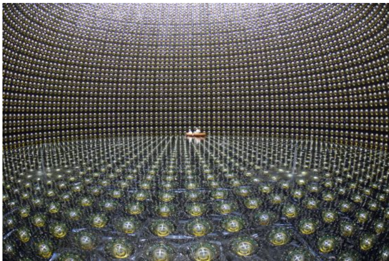
Interior del Super Kamiokande. Hyper Kamiokande será 20 veces mayor / KAMIOKA OBSERVATORY
